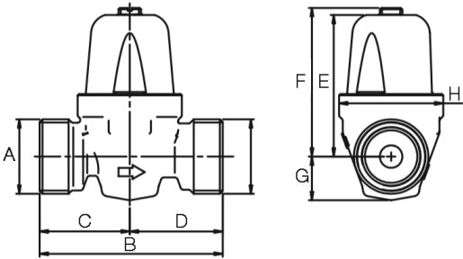
Multi-fileté Mâle 3/4" et Femelle 1/2" à l'entrée et la sortie
