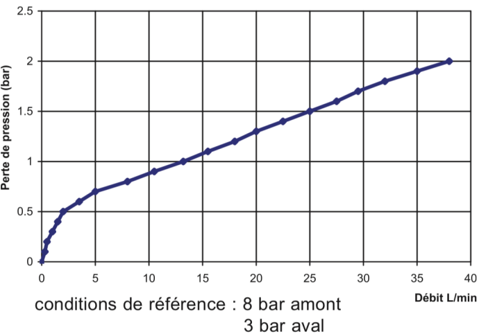
RÉDUBAR - Courbe de perte de charge
